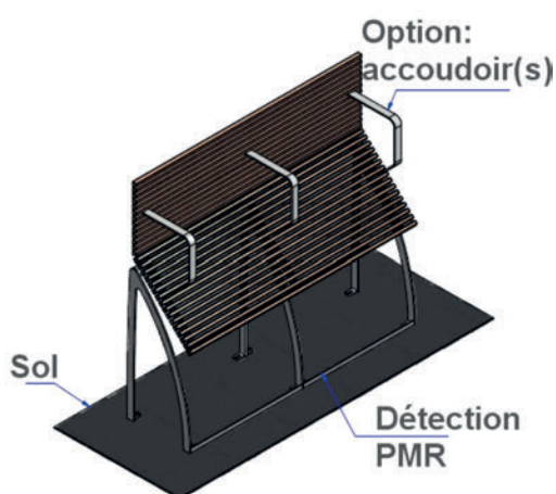
Assis-debout avec accoudoirs et détectable par les personnes aveugles et malvoyantes (source : Actus Mobilier urbain)
